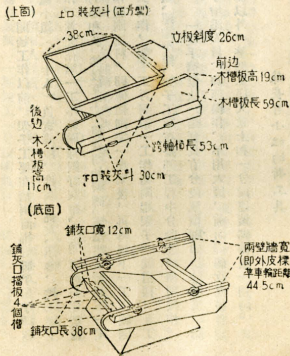
鋪灰器圖解
